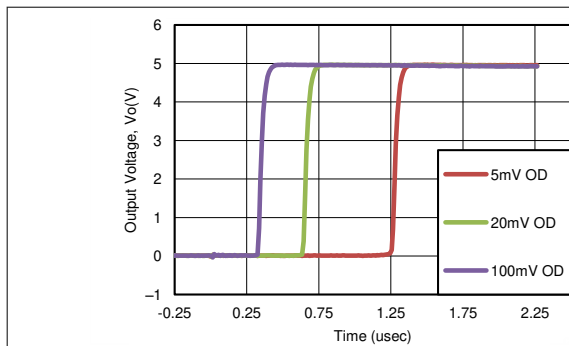
图 8-2. 各种过驱的响应时间 (正转换)
